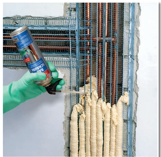
Dämmung von Heizrohren gegen Wärmeverluste.
