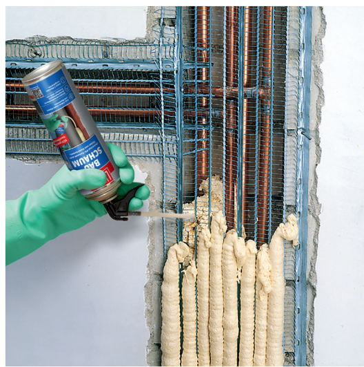
Dämmung von Heizrohren gegen Wärmeverluste.
