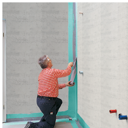
Einbetten von DICHTUNGSBAND in DUSCHABDICHTUNG in den Eckfugen.
