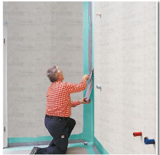
Einbetten von DICHTUNGSBAND in DUSCHABDICHTUNG in den Eckfugen.
